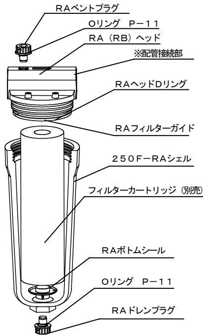
【構造 (RA・RB共通)】
