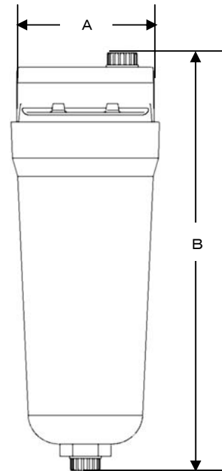
【寸法図 (数値は下表参照)】
