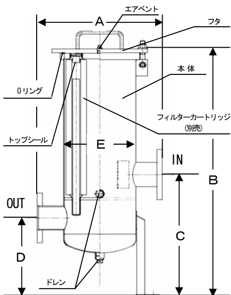
【構造 (SMC-750-6-*F)】
